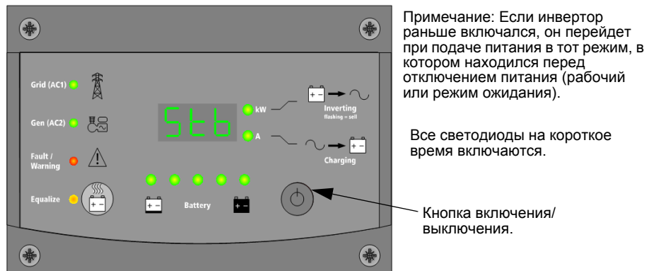
Рис. 2-17 Состояние дисплея при включении питания
