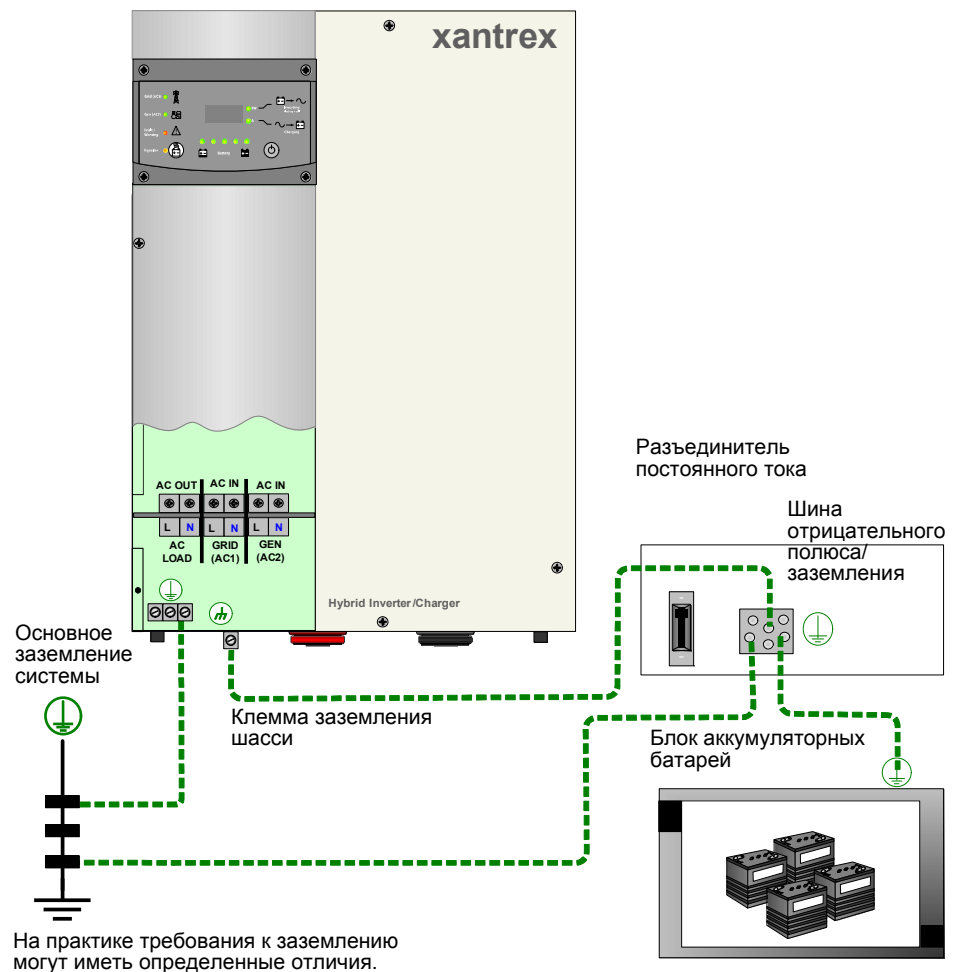
Рис. 2-8 Заземление по постоянному току с использованием силового распределительного щита
