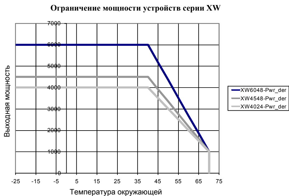
Рис. А-2 Зависимость выходной мощности от температуры окружающей среды
