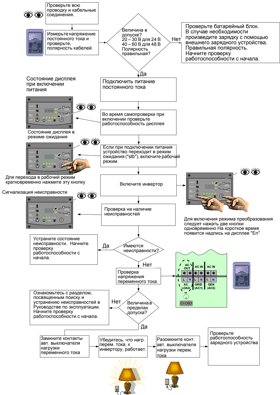
Рис. 2-21 Проверка работоспособности систем с одним инвертором
