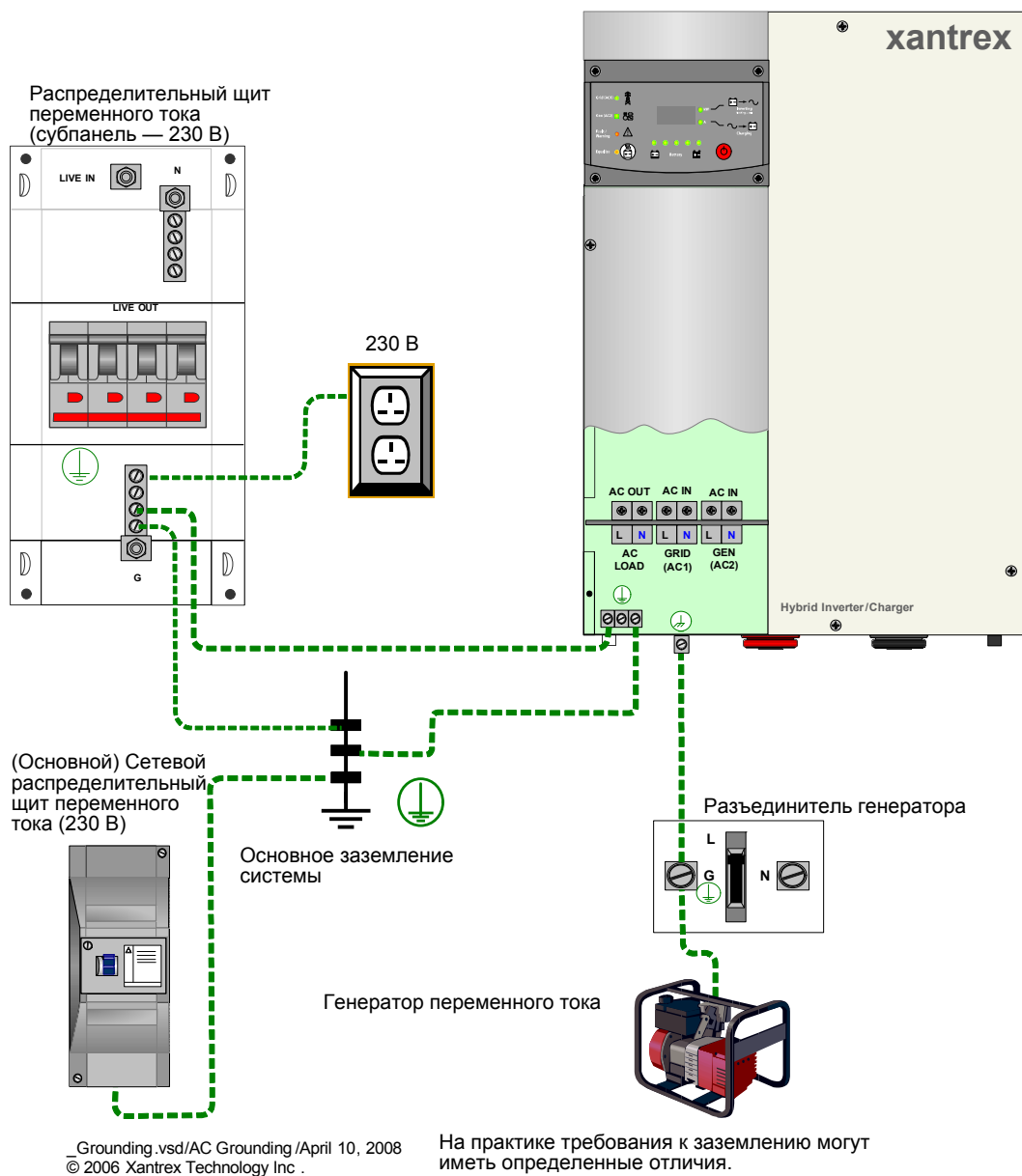
Рис. 2-13 Заземление системы переменного тока
