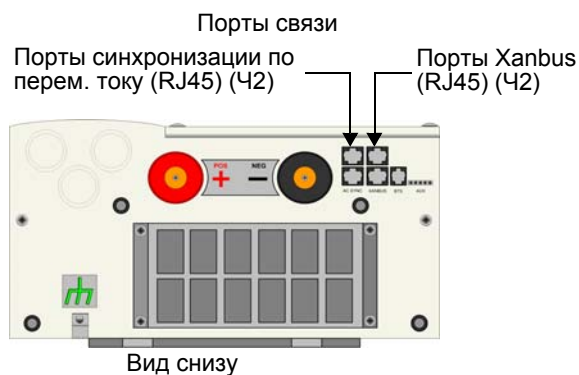
Рис. 2-5 Порты связи XW инвертора/зарядного устройства
