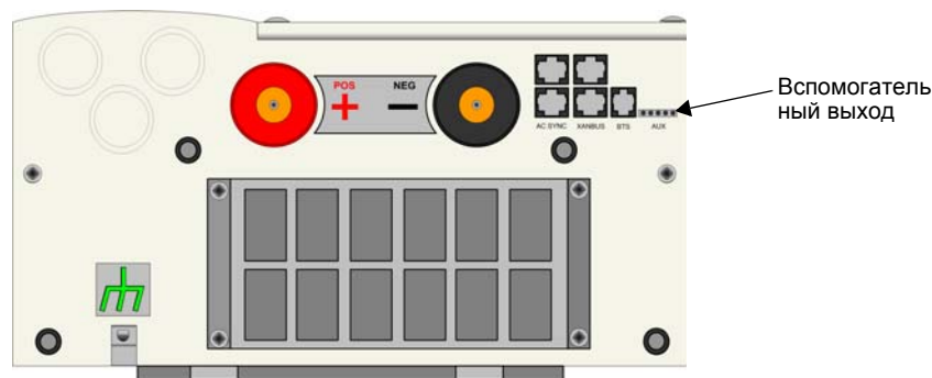
Рис. 2-16 Расположение вспомогательного выхода
