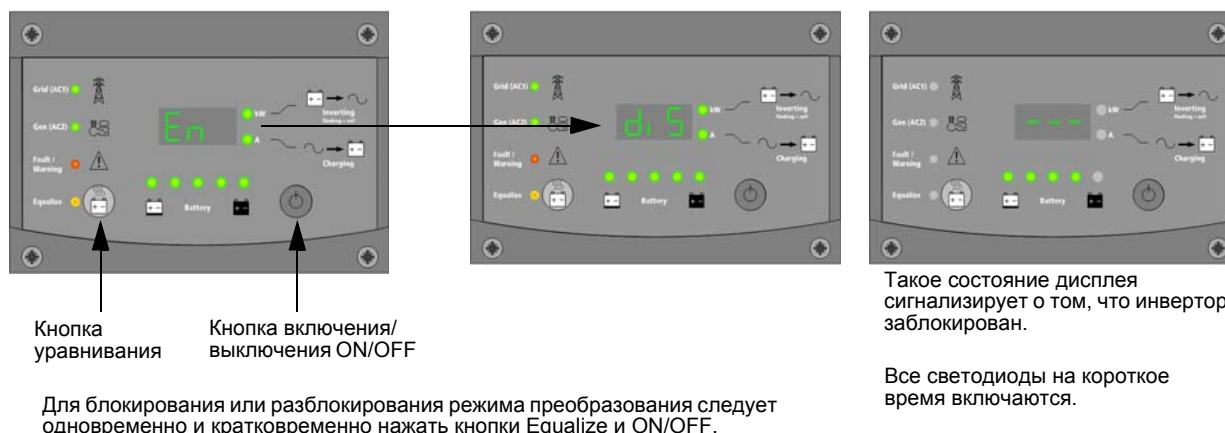
Рис. 2-18 Включение инвертора
