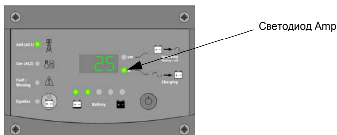
Рис. 2-20 Проверка режима зарядки батареи
