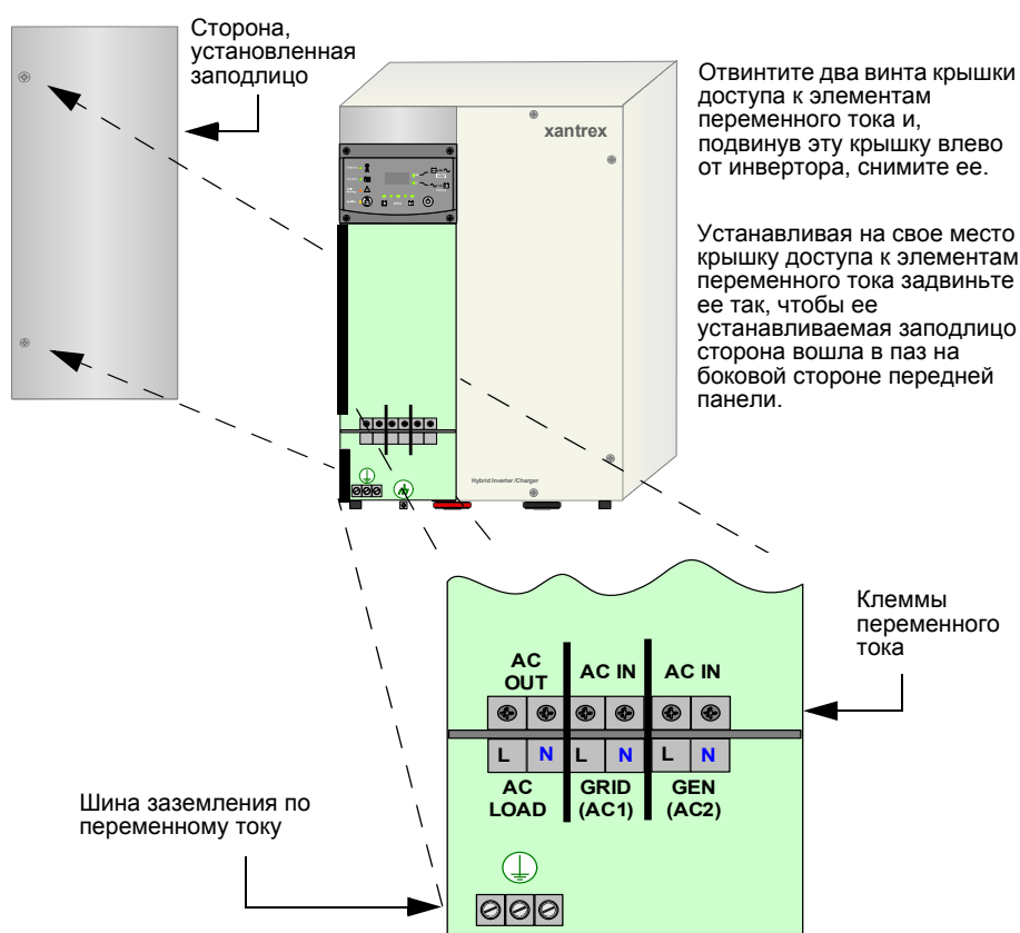
Рис. 2-12 Клеммная колодка переменного тока и шина заземления
